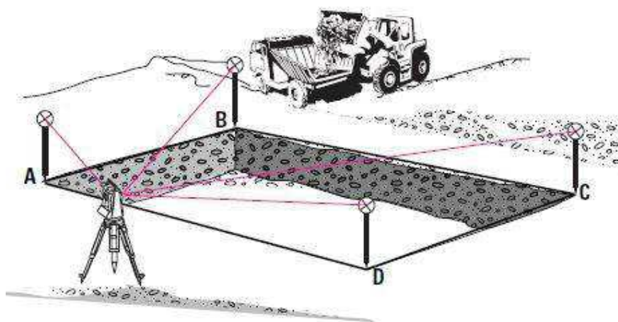
Figura 03 – Aplicação do método área
