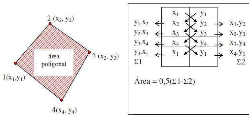
Figura 04 – exemplo de tabela para cálculo da área
