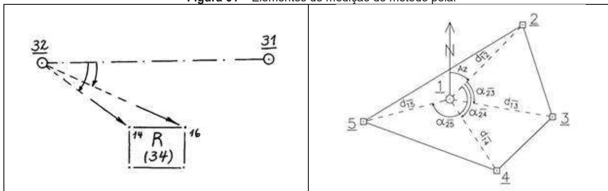
Figura 01 – Elementos de medição do método polar
