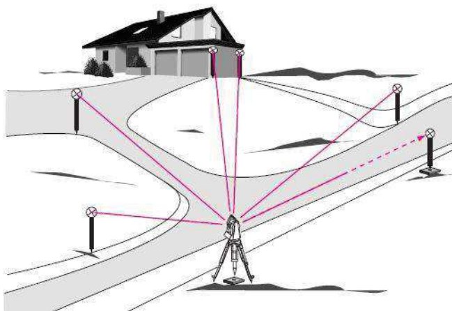
Figura 02 – Medição pelo método polar
