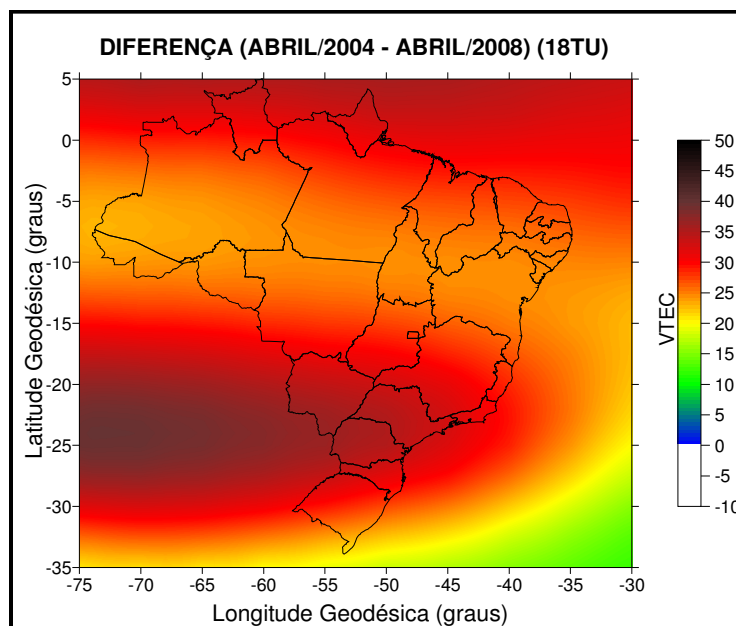
Figura 7. Mapas de diferenças de VTEC entre os meses de abril/2004 e abril/2008. Fonte: Penha (2009).
