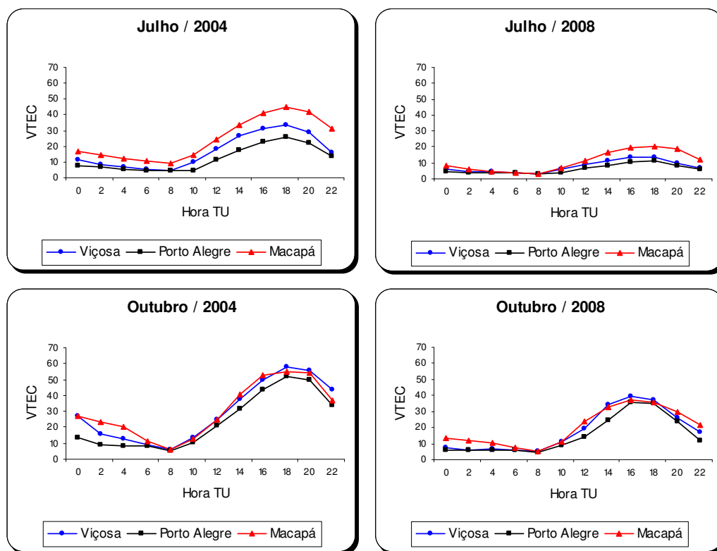
Figura 6. Valores médios mensais do VTEC para Viçosa, Porto Alegre e Macapá (julho/2004, outubro/2004, julho /2008 e outubro/2008).
