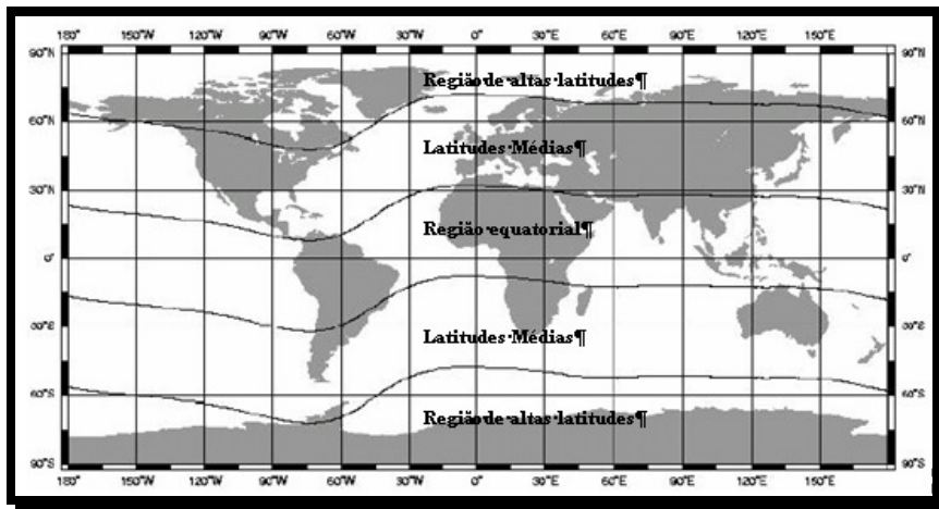
Figura 3. Regiões geográficas da ionosfera.
