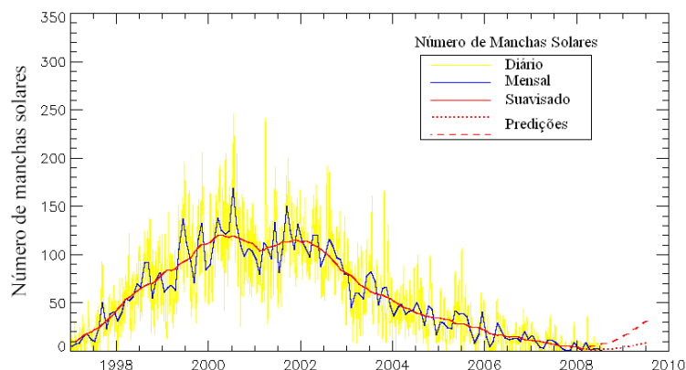
Figura 2. Ciclos solares 23 e 24.
