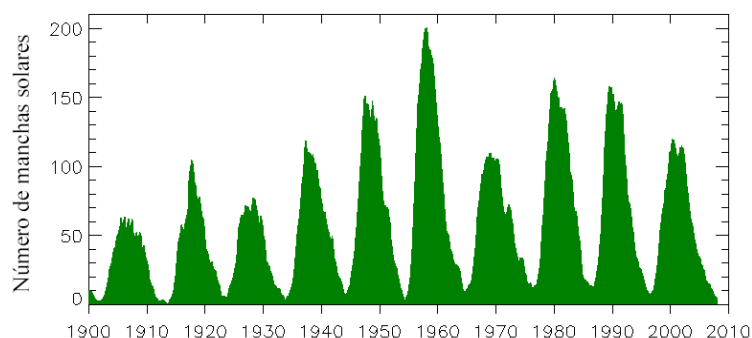
Figura 1. Número de manchas solares e ciclos solares.
