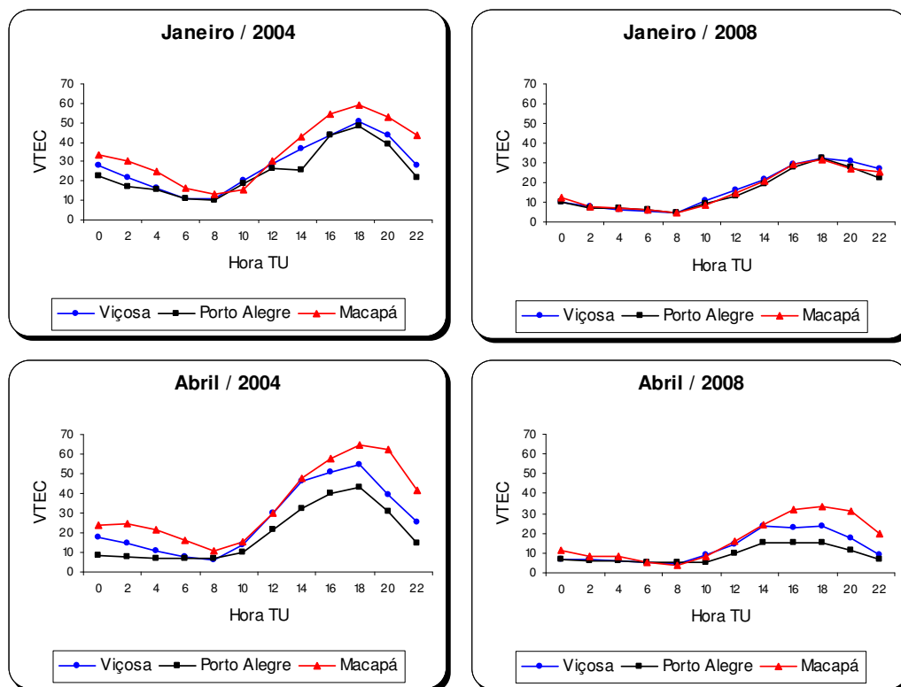
Figura 5. Valores médios mensais do VTEC para Viçosa, Porto Alegre e Macapá (janeiro/2004, abril/2004, janeiro/2008 e abril/2008).
