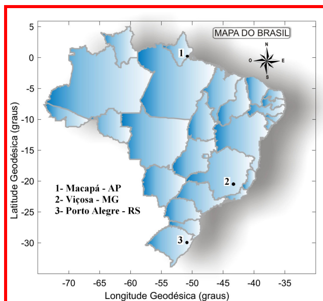
Figura 4. Localização da área de estudo.
